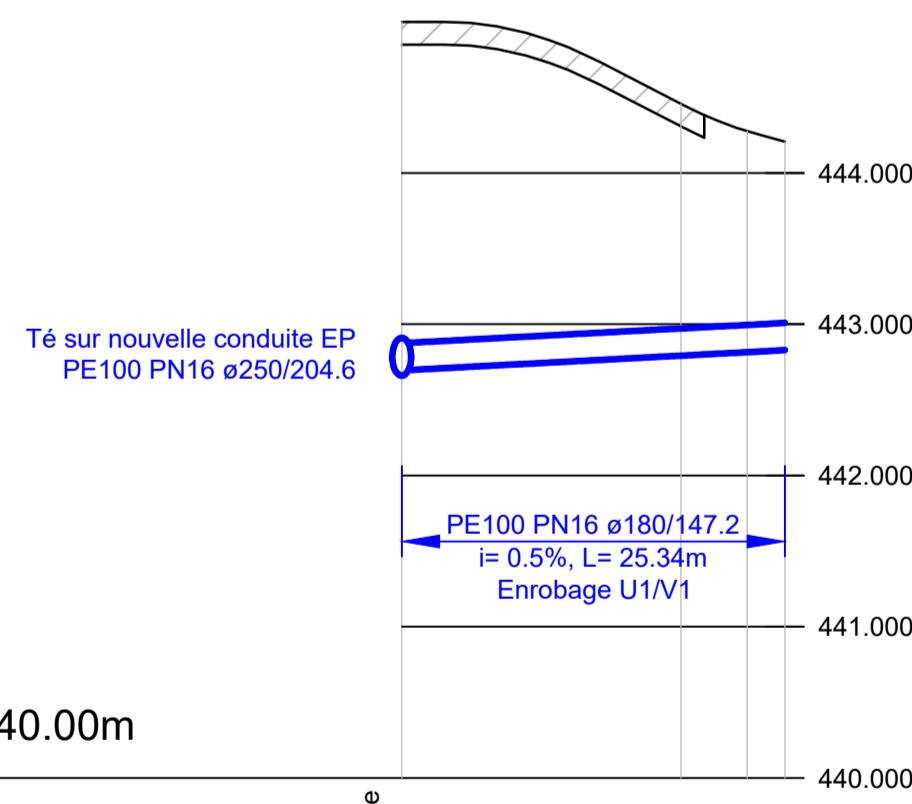
PROFIL EN LONG vers BH 33 1:500/50
